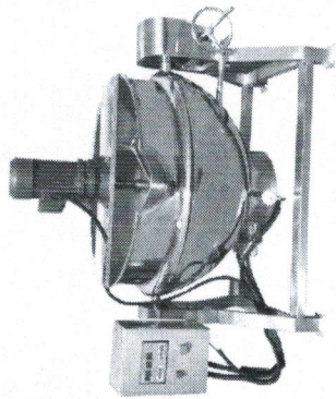
7. Машина для смешивания фруктов для приготовления фруктового джема.
