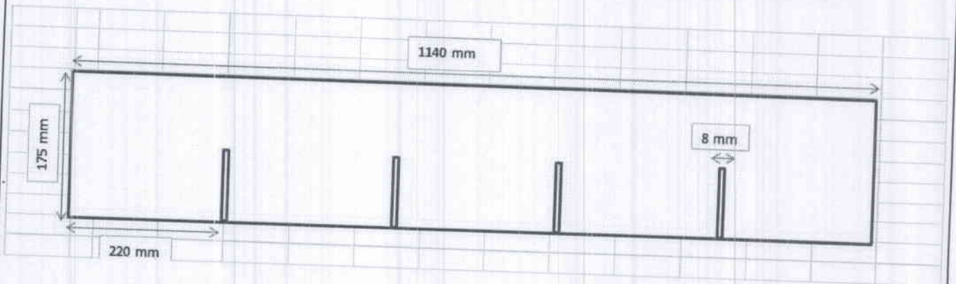
Дамас для передних фонарей решетка 1140*175 мм картонная с весом 0,100 кг тип ПЗ2ВС
