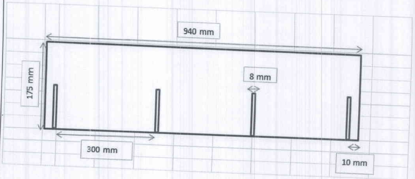
Дамас для передних фонарей решетка 940*175 мм картонная с весом 0,100 кг тип ПЗ2ВС
