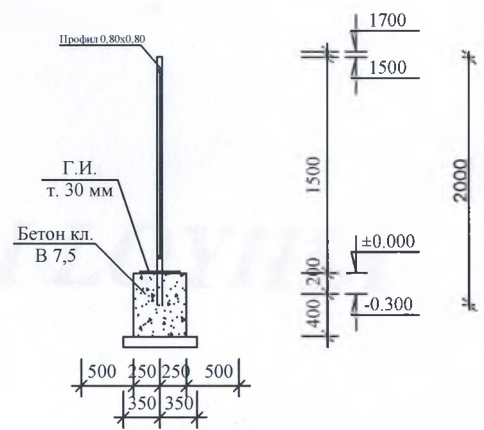
Разрез 2 - 2
