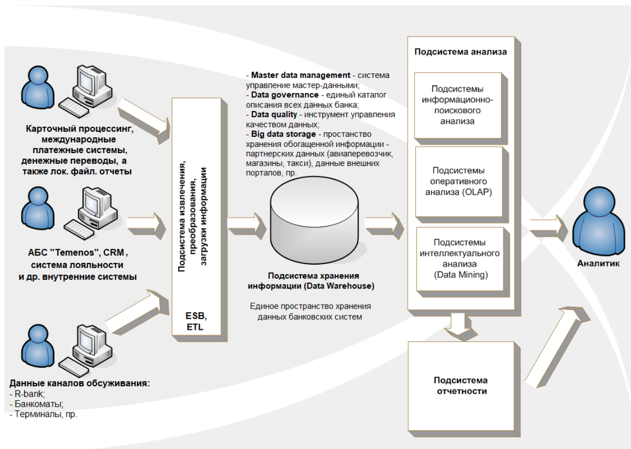
Рис.2 Схема потоков данных Корпоративного хранилища данных
