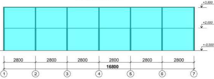
План теплицы
