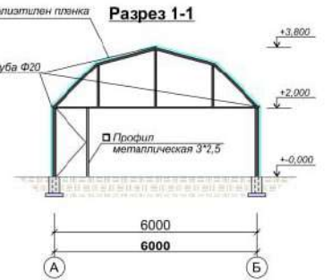
Разрез 1-1
