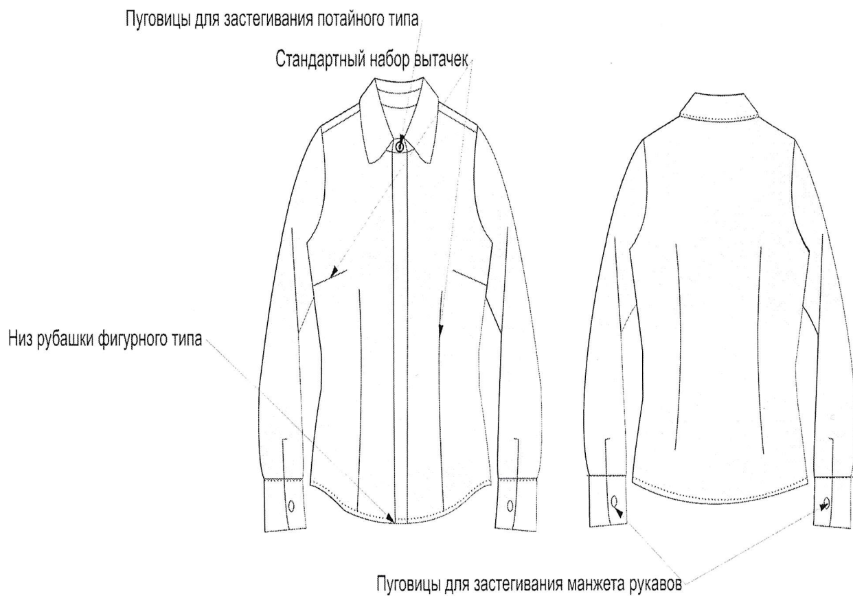
Рис.1 Технический рисунок Блузки
