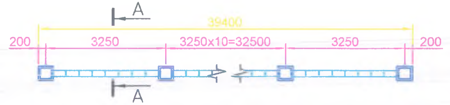
Фрагмент плана ограждения. ОГ-2
