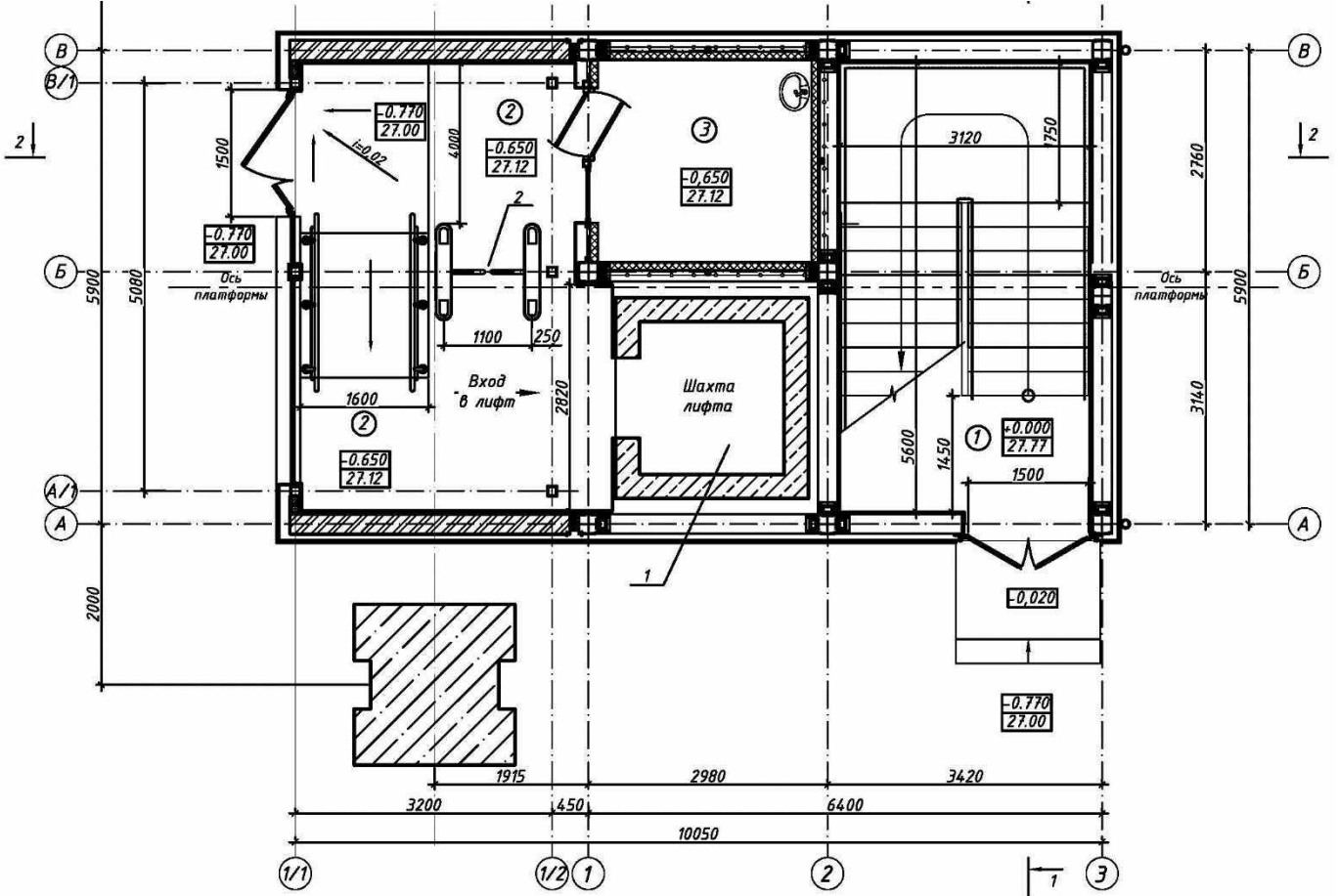
Чертеж №1/1 (Вход для людей с ограниченными возможностями станциях от №8 до №12)
