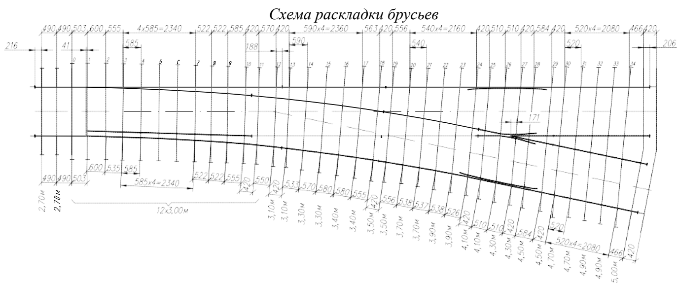
Рисунок 1. Стрелочный перевод типа Р65 марки 1/5 ВСП06.00.0000
