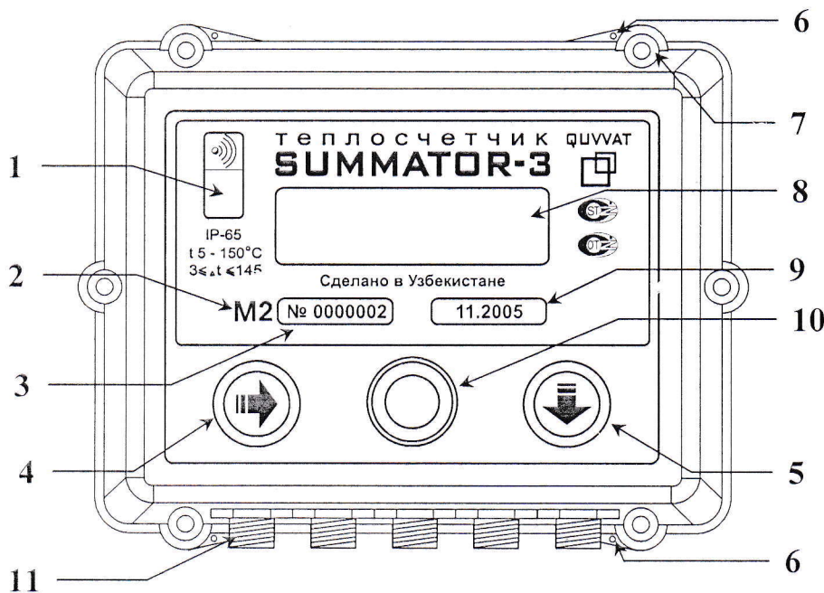
Рисунок 1 (вид спереди)
