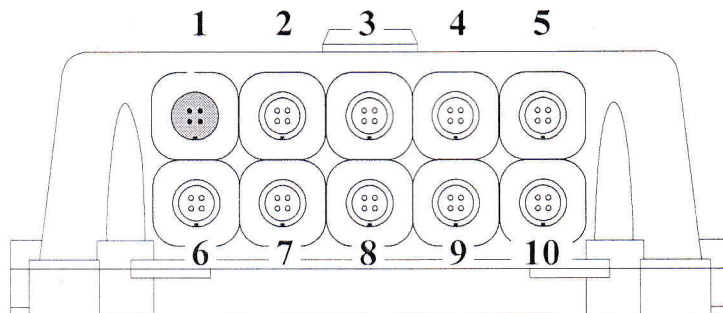
Рисунок 2 (разъемы, вид снизу)
