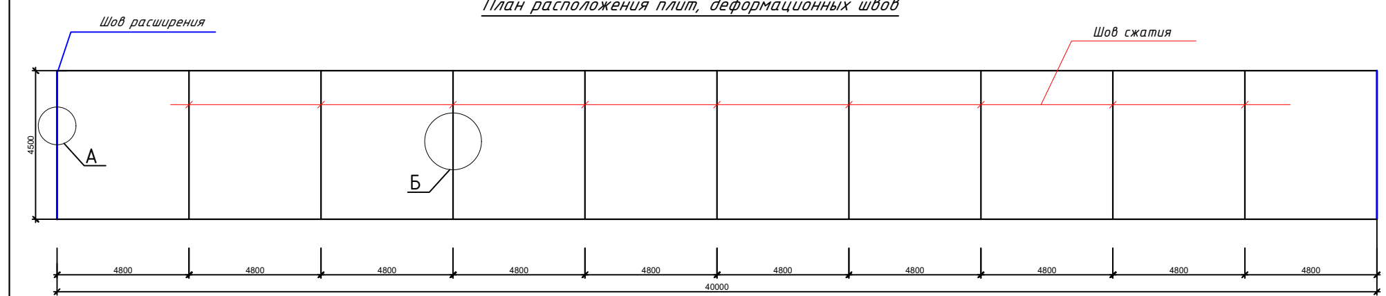
План расположения плит, деформационных швов
