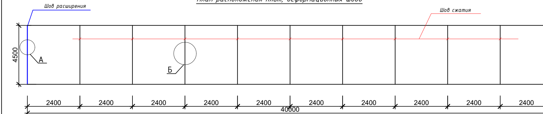
План расположения плит, деформационных швов
